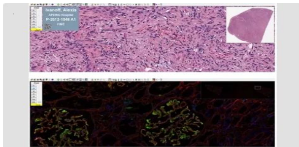
Aperio ImageScope
