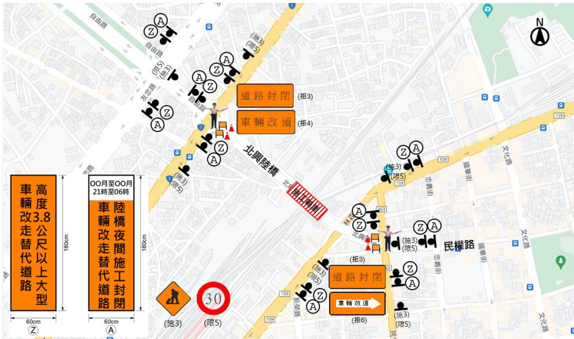
施工期間北興陸橋相關施工設施佈設示意圖
