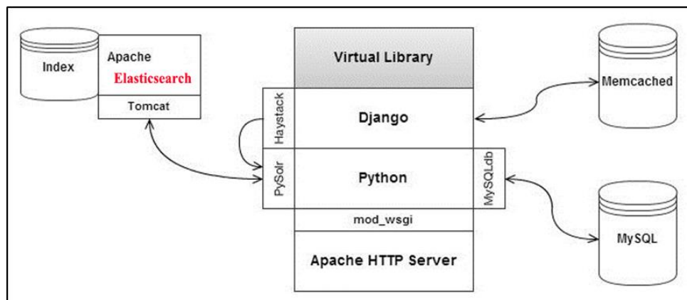
圖十、全新打造的資訊安全檢測系統架構
