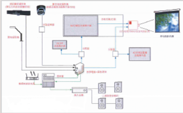
母系206數位學習教室系統配置圖
